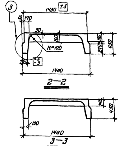
СПЕЦИФИКАЦИЯ МАРКИ ЭЛЕМЕНТОВ НА ОДНУ ПЛИТУ
